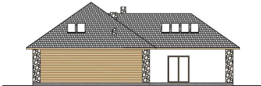
ELEWACJA TYLNA
