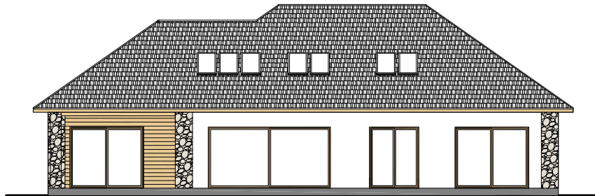
ELEWACJA BOCZNA
