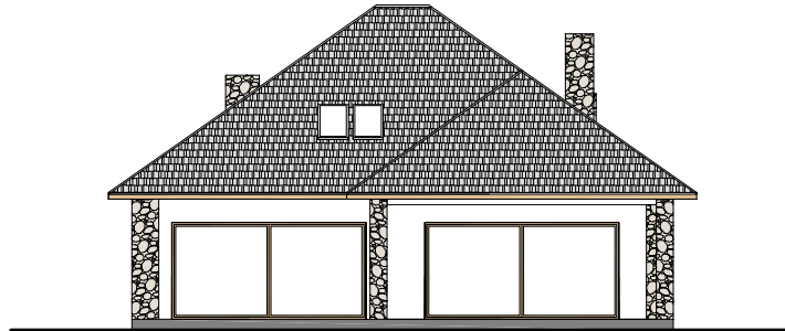
ELEWACJA TYLNA
